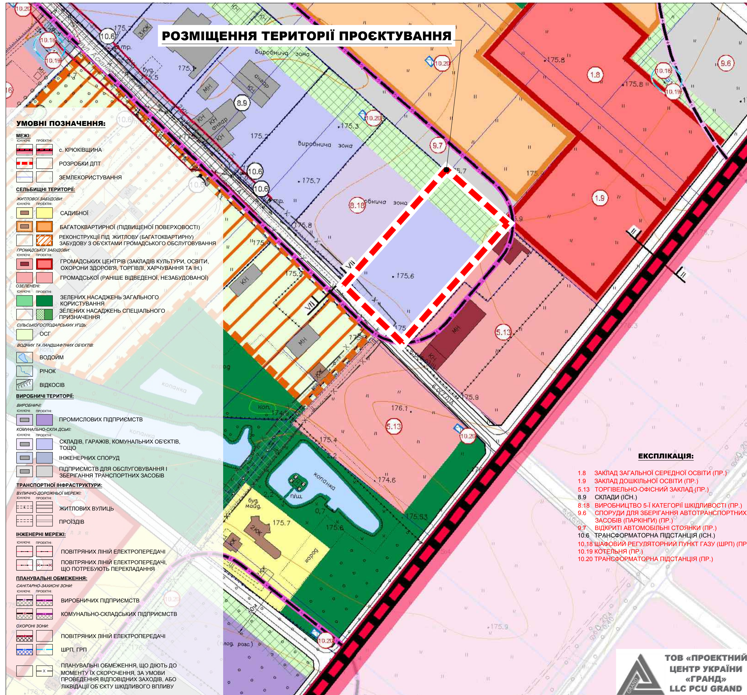
СХЕМА РОЗТАШУВАННЯ ТЕРИТОРІЇ ДЕТАЛЬНОГО ПЛАНУ ТЕРИТОРІЇ В СИСТЕМІ ПЛАНУВАЛЬНОЇ СТРУКТУРИ ТЕРИТОРІАЛЬНОЇ ГРОМАДИ
